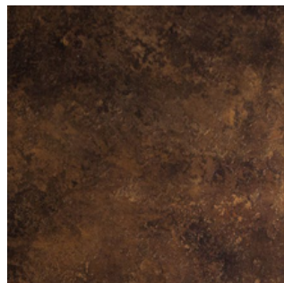
Limonite d'Eau
